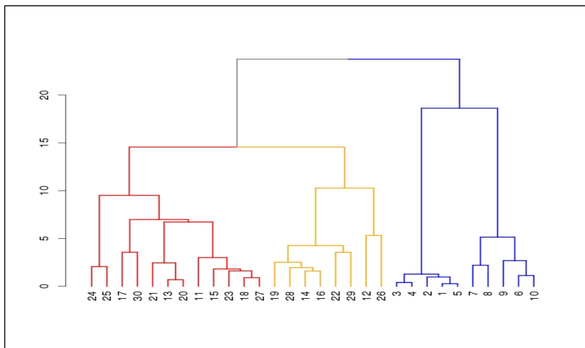
Gráfico 3.1: Exemplo de dendrograma.
